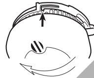
FIG 3. (MODÈLE LL UNIQUEMENT), POUR DÉTACHER UN DÉTECTEUR DE SA PLATE-FORME DE MONTAGE, POUSSEZ CETTE PARTIE VERS LE HAUT AVEC UN PETIT OUTIL, PUIS FAITES PIVOTER LE DÉTECTEUR-AVERTISSEUR DANS LE SENS DES AIGUILLES D'UNE MONTE
